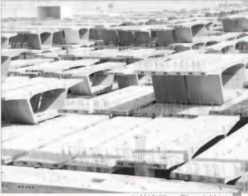
إعداد قطع الجسور والتأكد من موائمتها قبل تركيبها
