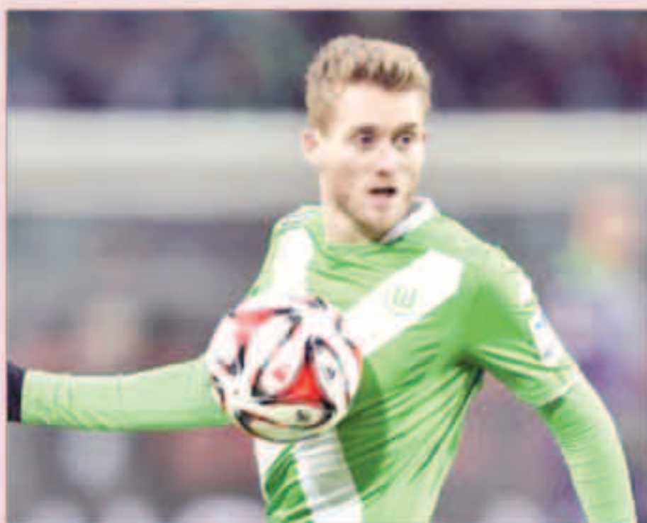
تبدیل شوریه
