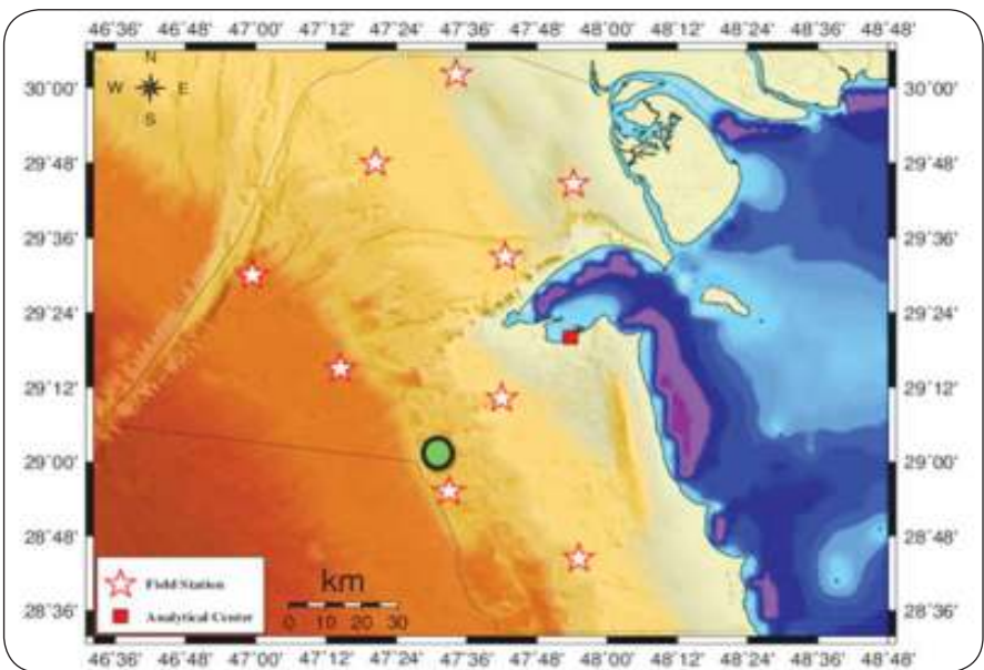
موقع زلزال الكويت في الخريطة
