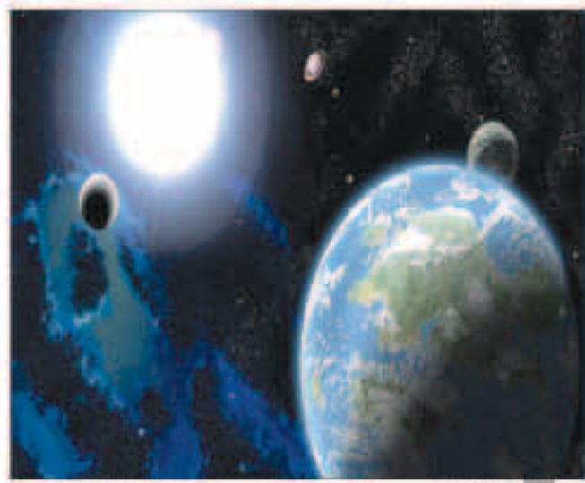
ثلاثة كواكب بحجم الأرض يمكن أن تضم محيطات مياه سائلة
