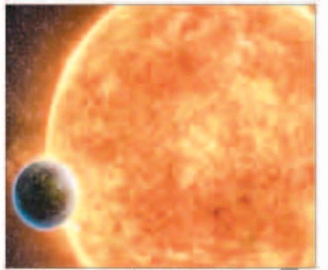
رسم يظهر الأرض السوبر قرب نجمها
