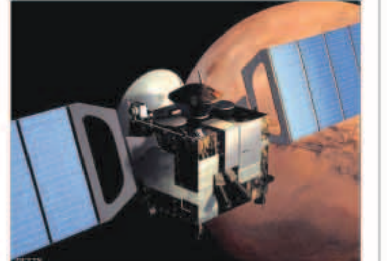
تسجيل سلسلة من النبضات المغناطيسية الغامضة على المريخ
