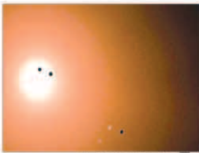
عطارد سيبدو كنقطة سوداء في قرص الشمس
