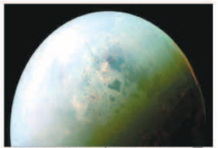
«تيتان» يبلغ طول قطره 5150 كيلومتراً، هو ثاني أكبر قمر في المجموعة الشمسية
