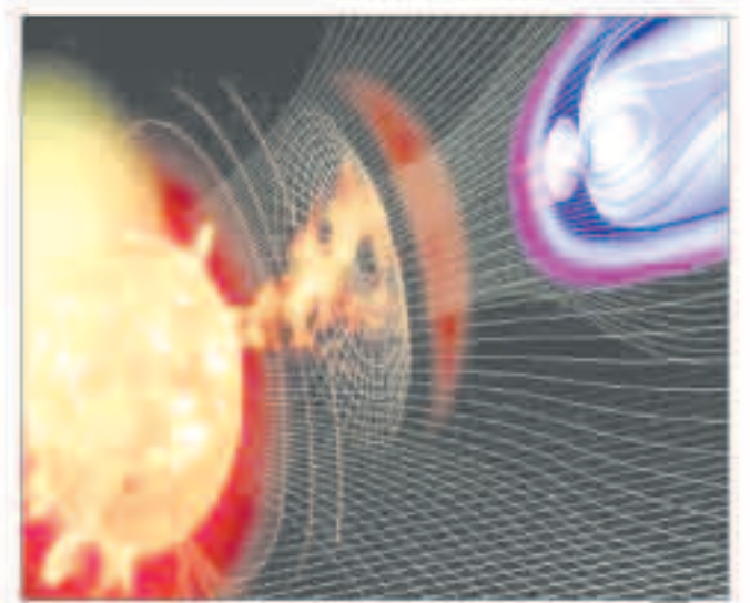
إحدى العواصف الشمسية من وكالة الفضاء الأمريكية (ناسا)
