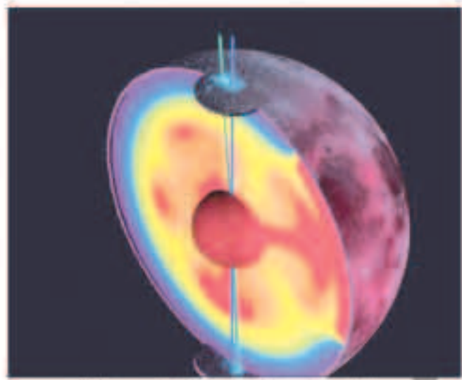
رسم فناني نظرية مجموعة «نيشتر» يظهر كيفية تغير محور دوران القمر
