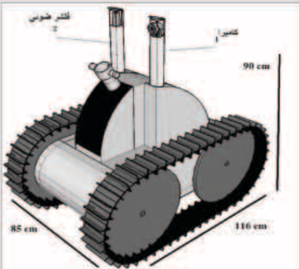
صورة الروبوت لمكافحة الحرائق
